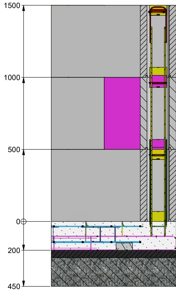
A-A ( 1 : 15 ) gedreht um 90°
