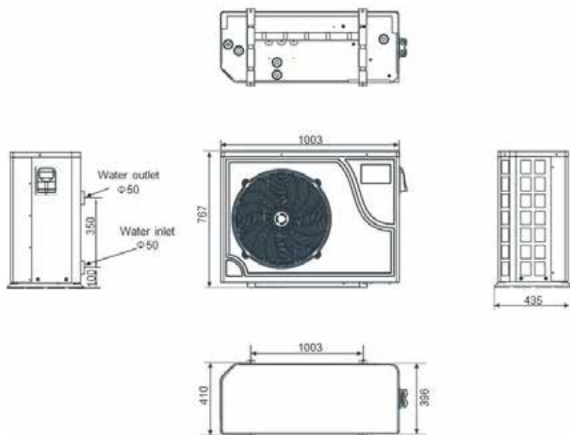
Abmaß Schwimmbad-Wärmepumpe »SUPERIOR 12« in mm
