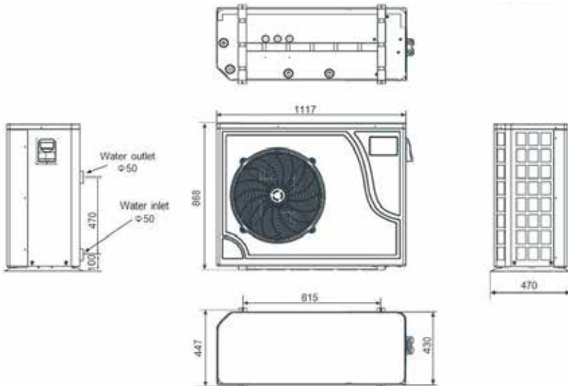
Abmaß Schwimmbad-Wärmepumpe »SUPERIOR 17« in mm
